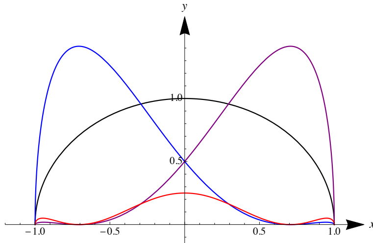
Слика 2.2: Графици тежинских функција x \mapsto w(x) , x \mapsto \tilde{w}(x) , x \mapsto \bar{w}(x) и x \mapsto \hat{w}(x) на интервалу [-1, 1]
