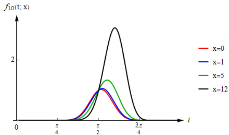
Слика 5.6: Графици интегранда t \mapsto f_{10}(t; x) у интегралу Q_{10}^1(x) , t \in (0, \pi) за x = 0, 1, 5 и 12
