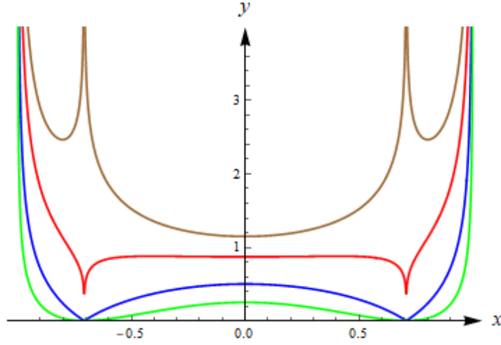
Слика 3.1: Графици тежинске функције x \mapsto w^{2,s}(x) на (-1, 1) , за s = -1/10 (браон линија), s = 1/10 (црвена линија), s = 1/2 (плава линија) и s = 1 (зелена линија)
